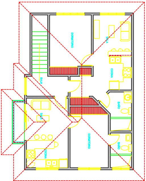
PLANTA DE DISTRIBUCION ARQUITECTONICA 4° NIVEL ESCALA 1: 50
